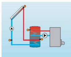
Sistem solar de productie apa calda menajera si cu aport la incalzire
