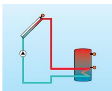
Sistem solar de productie apa calda menajera
